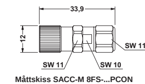
Måttskiss SACC-M 8FS-...PCON
