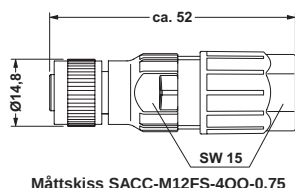
Måttskiss SACC-M12FS-4QO-0,75
