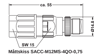
Måttskiss SACC-M12MS-4QO-0,75
