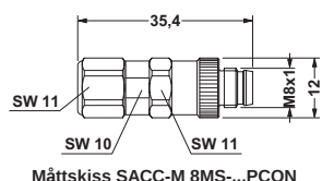
Måttskiss SACC-M 8MS-...PCON
